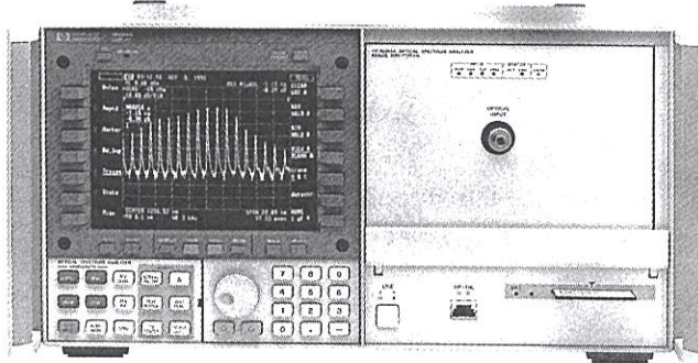
HP 71450A
