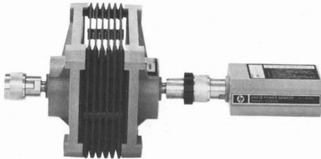
HP 8481B
